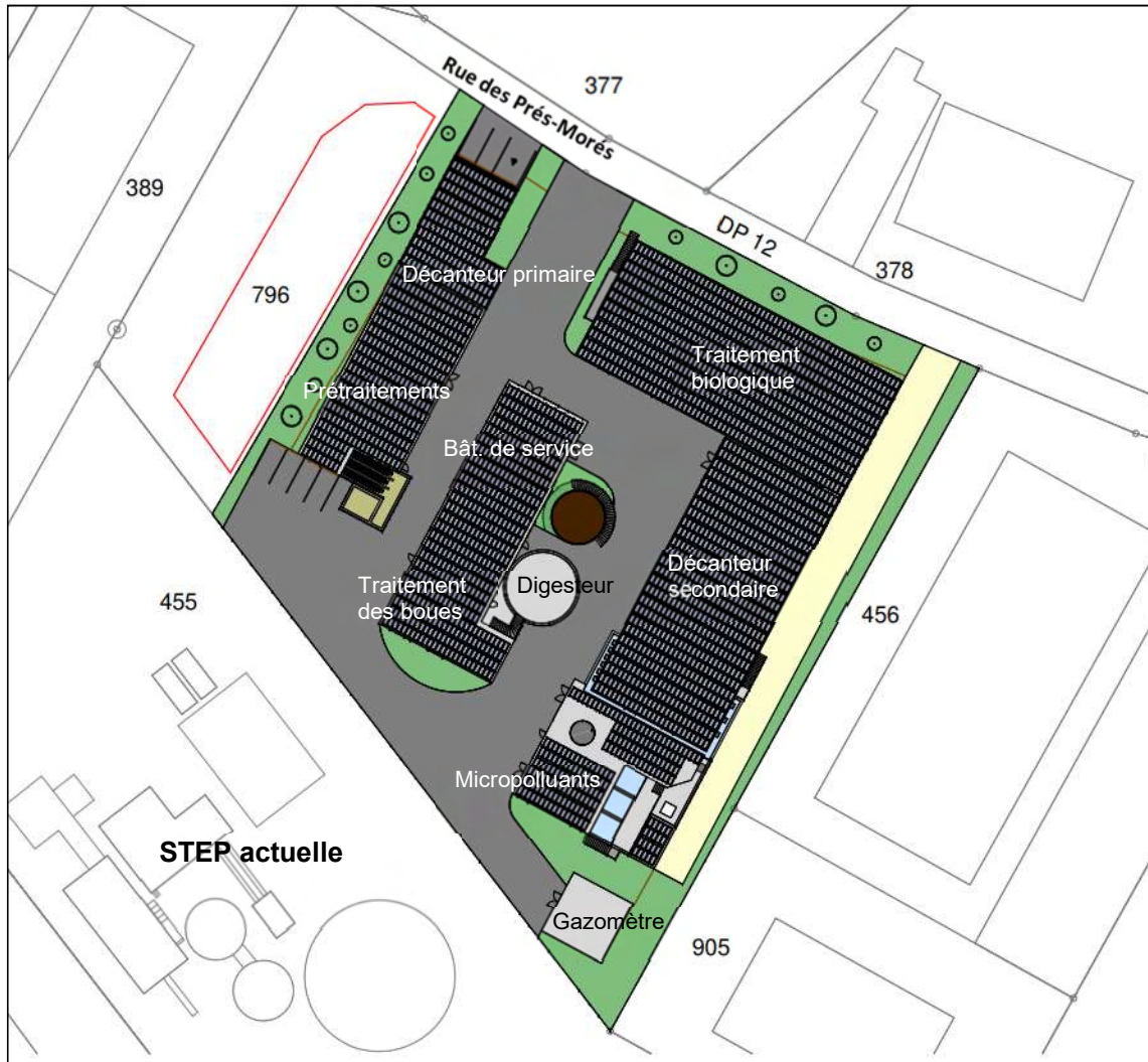
Figure 2: Plan de situation de l'avant-projet de STEP régionale sur le site de La Sarraz
