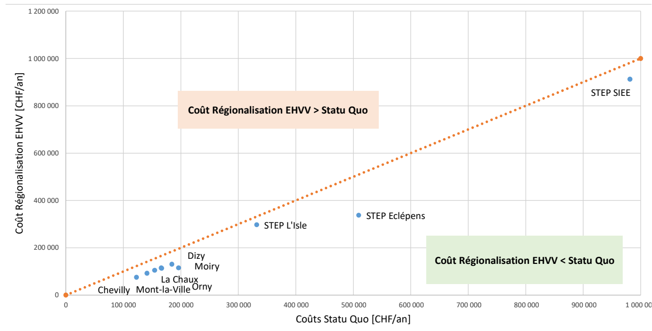
Figure 4 : Comparatif entre les coûts totalisés par STEP (charges financières et charges d'exploitation) du Statu quo (renouvellement et mise aux normes des 10 STEP existantes) (axe horizontal) par rapport à la Régionalisation (axe vertical). Chaque point représente une STEP. Les STEP qui se situent sous la diagonale orange sont avantagées avec un projet régional.
